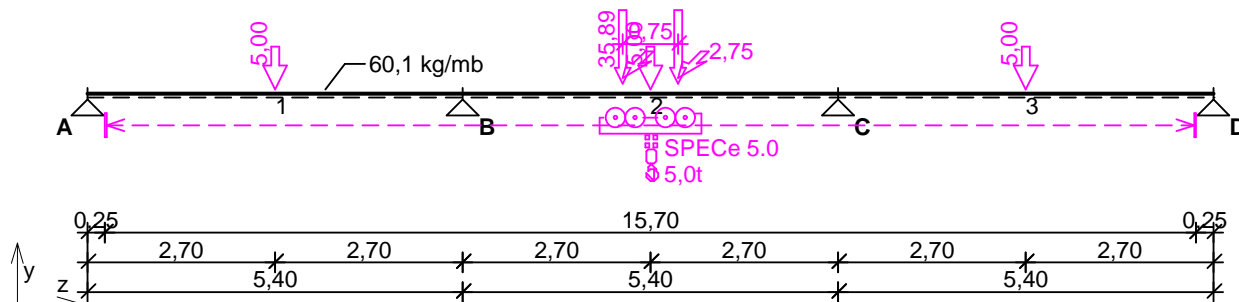
Tablica obciążeń obliczeniowych stałych (dodatkowo ciężar belki g_o = 0,65 \text{ kN/m} )
