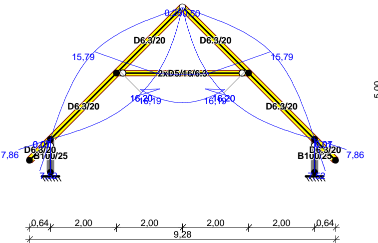
Obwiednia naprężeń:
